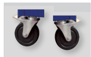
Rollen mit Roll- und Drehbremse Full Break System
