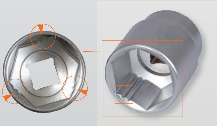
85% abgerundet / rounded
