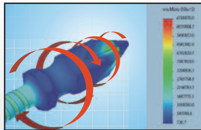
PROJAHN TORSION-Bit Kräfte werden in den Bit abgeleitet / Forces will disperse at torsion zone
