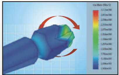
Standard-Bit Kräfte werden an der Spitze zentriert / Forces will accumulated at the tip of bit
