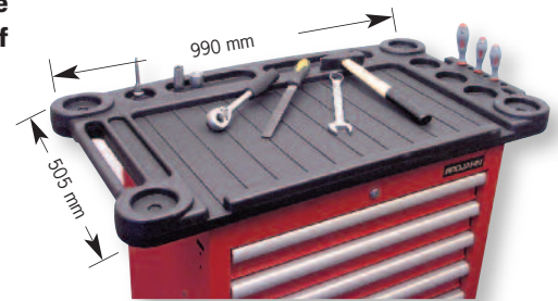
Arbeitsauflage aus Kunststoff Top Table
